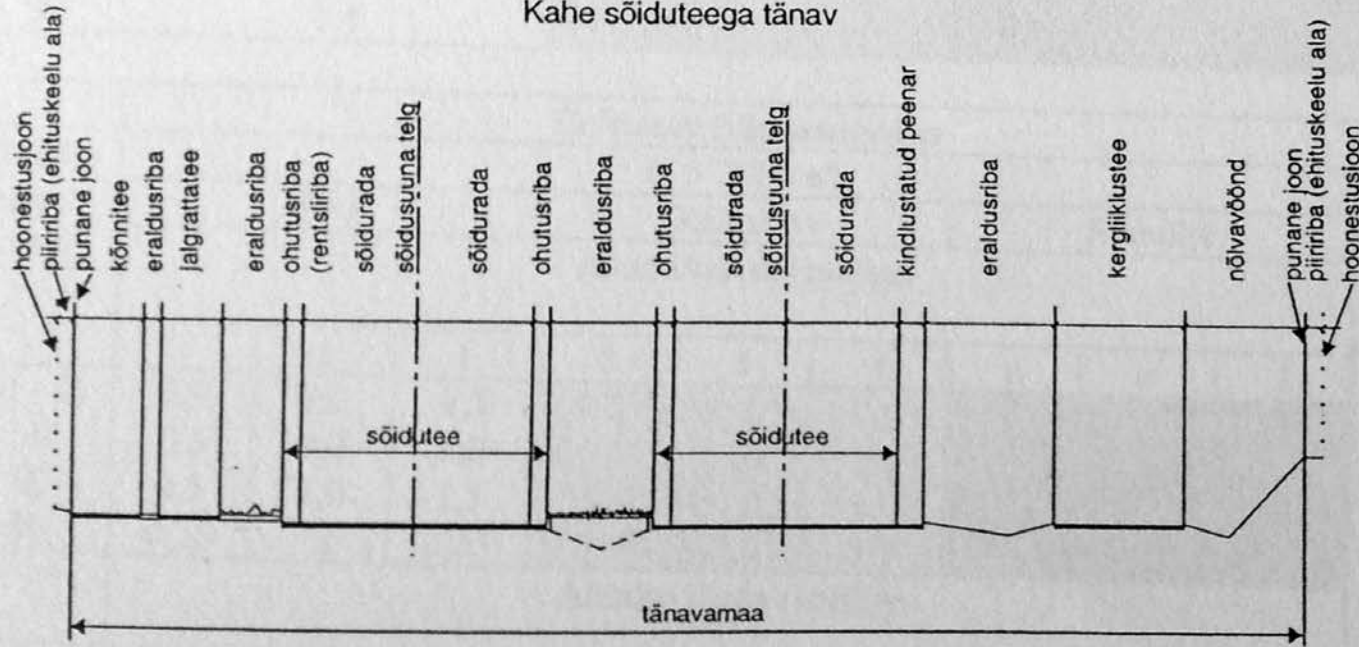
Joonis 7.1 - Tänav ristprofili võimalikud elemendid
